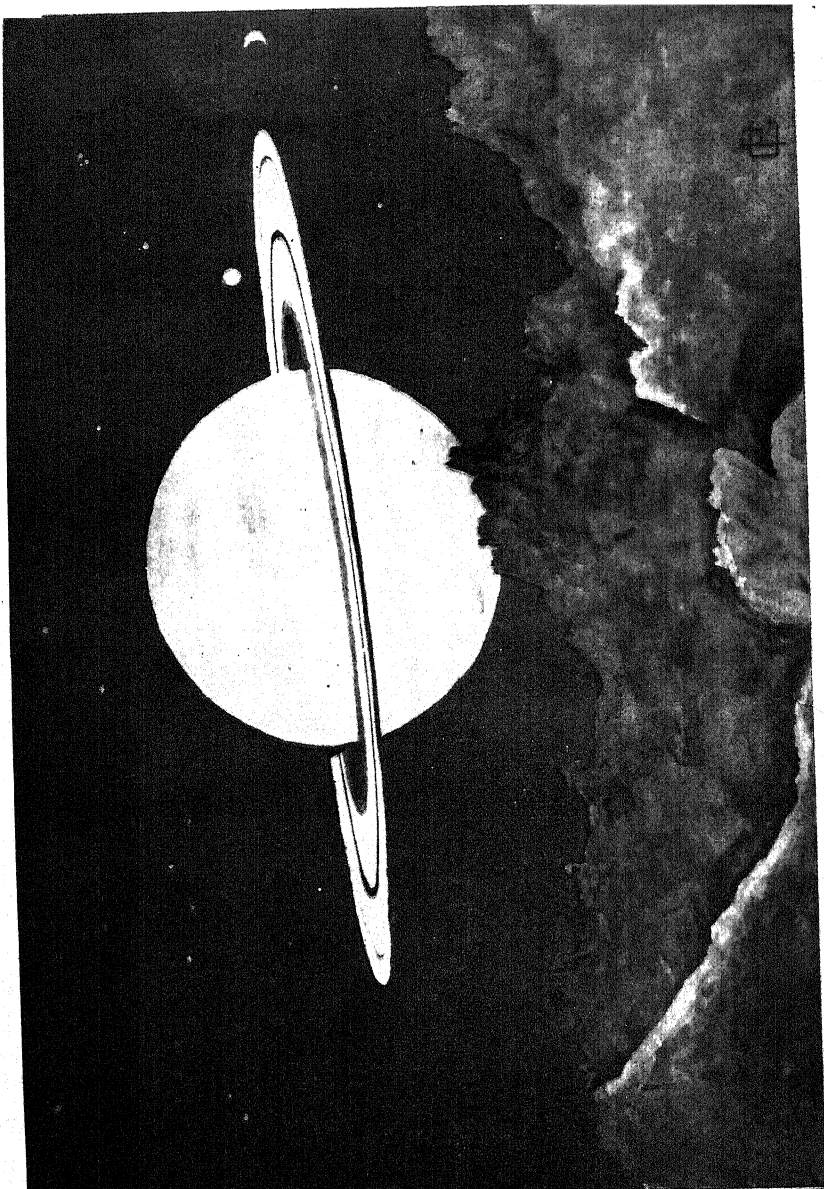
चित्र ३४—शनि के ही उपग्रह से शनि का एक काल्पनिक दृश्य इस में शनि के दो उपग्रह भी दिखाई पड़ रहे हैं। [ सौर-परिवार से ]
